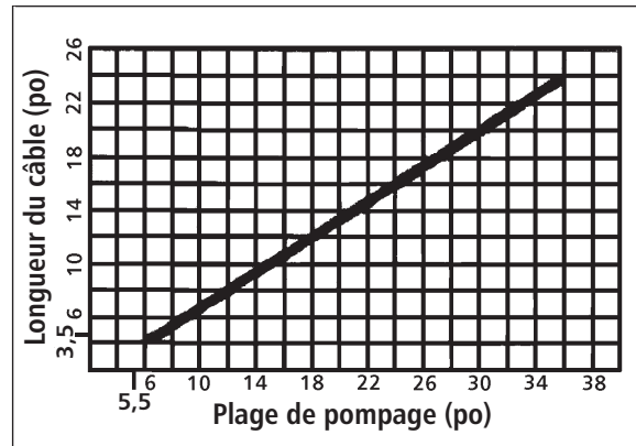
Courbe plage de pompage- longueur du câble
